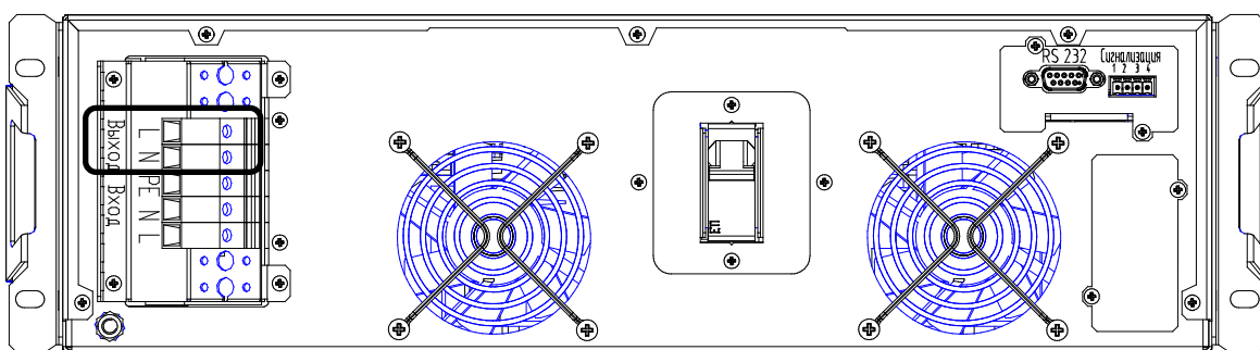
Рисунок 13а – Стабилизатор ИнСтаб IS1106RT, IS1108RT и IS1110RT. Выводы «Выход N-L»
