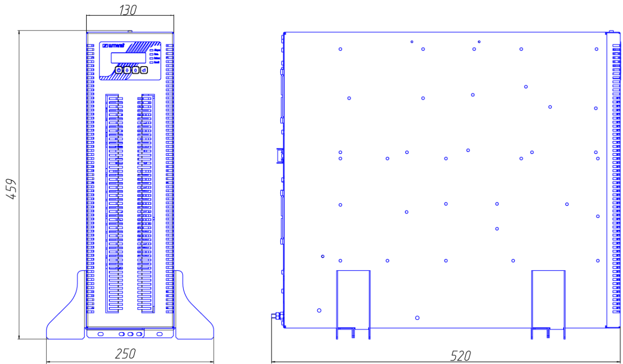
Рисунок 2а – Габаритные размеры стабилизаторов Штиль IS1106RT, IS1108RT, IS1110RT (напольное исполнение)
