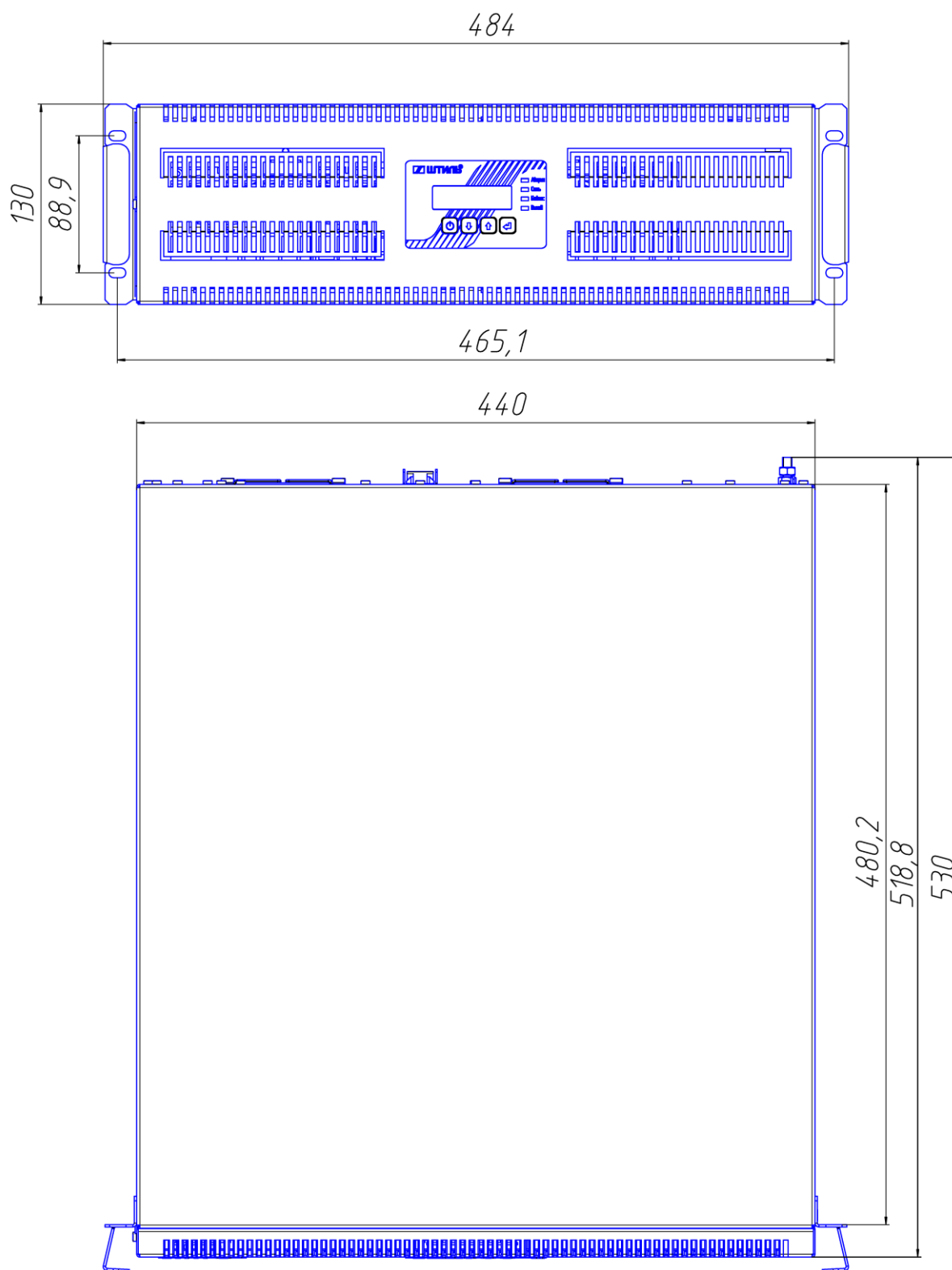
Рисунок 2в – Габаритные размеры стабилизаторов Штиль IS1106RT, IS1108RT, IS1110RT (стоечное исполнение)
