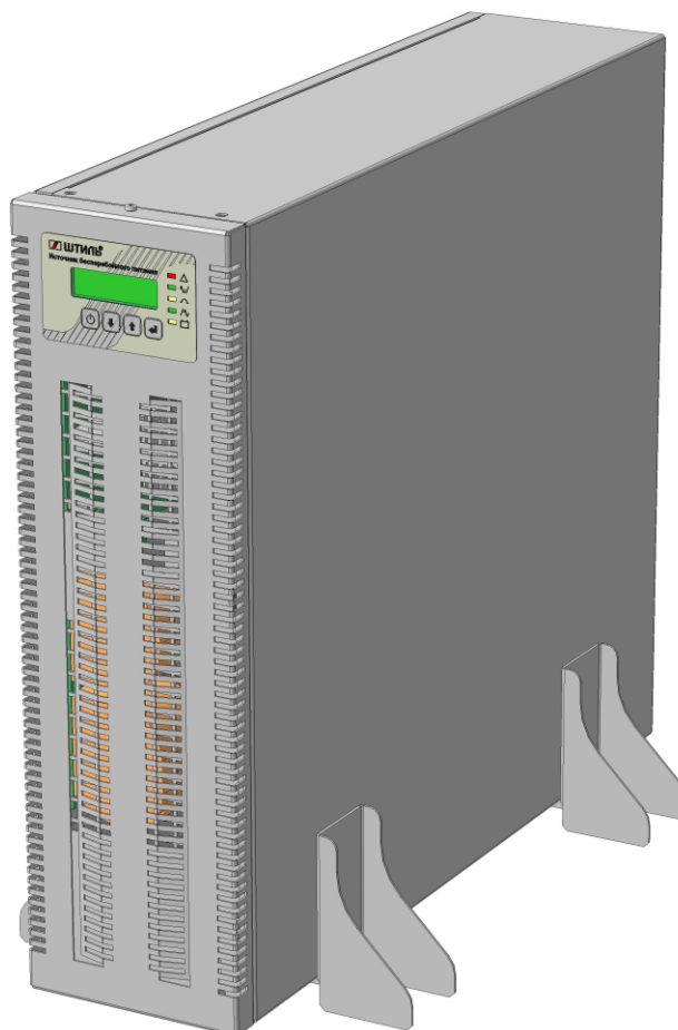
Рисунок 1б – Стабилизаторы Штиль IS1106RT, IS1108RT, IS1110RT (напольное исполнение)
