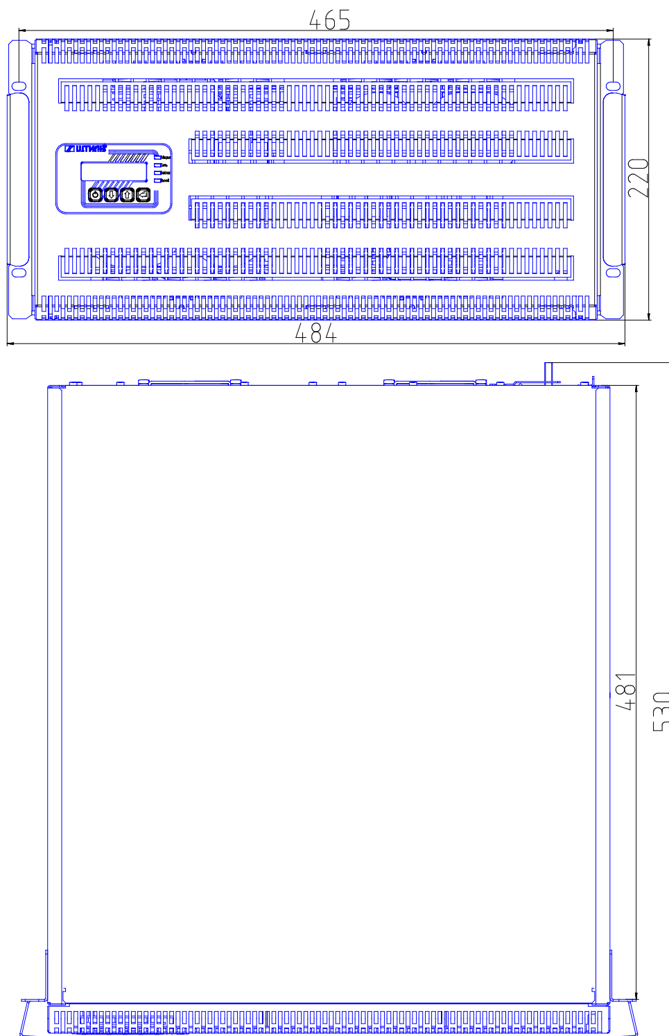
Рисунок 2Г – Габаритные размеры стабилизаторов «Штиль» IS1115RT и IS1120RT (стоечное исполнение)
