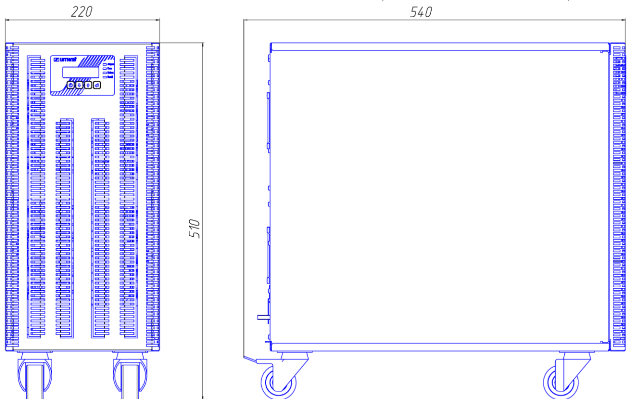
Рисунок 2б – Габаритные размеры стабилизаторов Штиль IS1115RT и IS1120RT (напольное исполнение)
