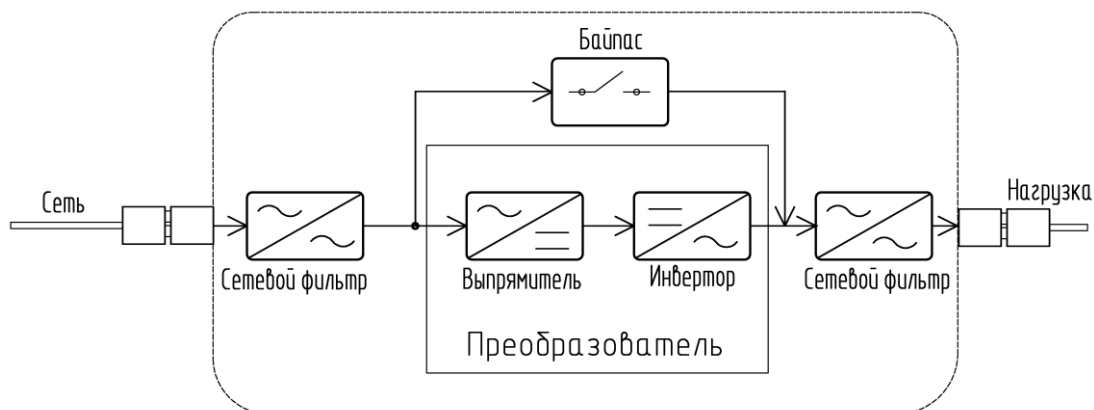
Рисунок 4 – Структурная схема принципа работы стабилизатора
