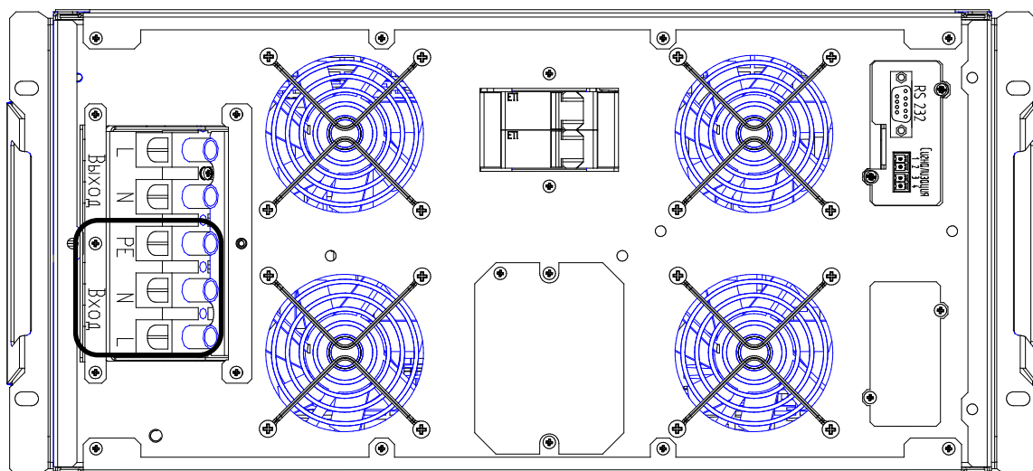
Рисунок 12б – Стабилизатор ИнСтаб IS1115RT и IS1120RT. Выводы «Вход PE-N-L»
