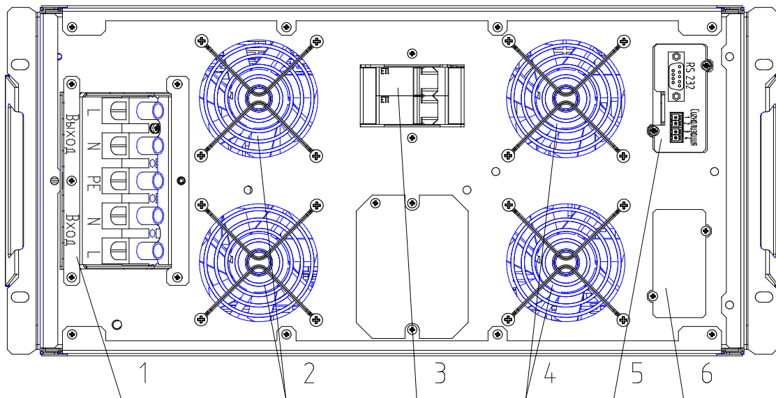
Рисунок 3а – Компоненты задней панели стабилизаторов Штиль IS1106RT, IS1108RT, IS1110RT
