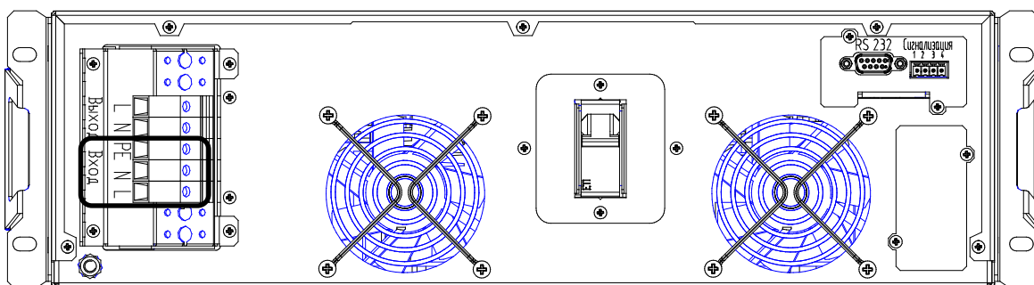
Рисунок 12а – Стабилизатор ИнСтаб IS1106RT, IS1108RT и IS1110RT. Выводы «Вход PE-N-L»
