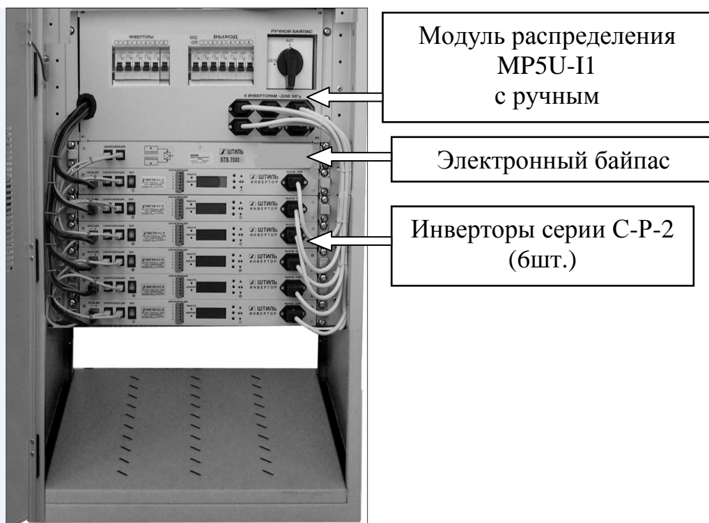
Рисунок 1.7 - Инверторная система мощностью 7,5 кВт с использованием модуля распределения MP5U-II и электронного байпаса STS 7500
