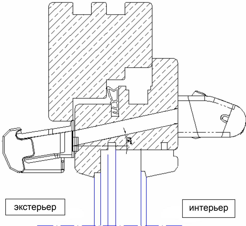
Рекомендуемые размеры технологического паза
